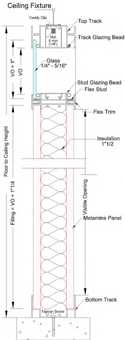
Detail A-A
