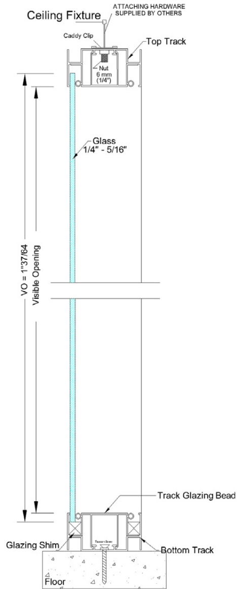
Detail A-A
