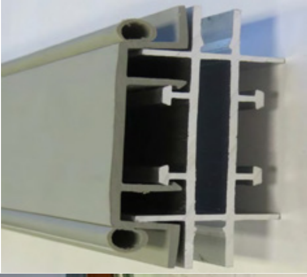
Stud bead snapping into a Stud
